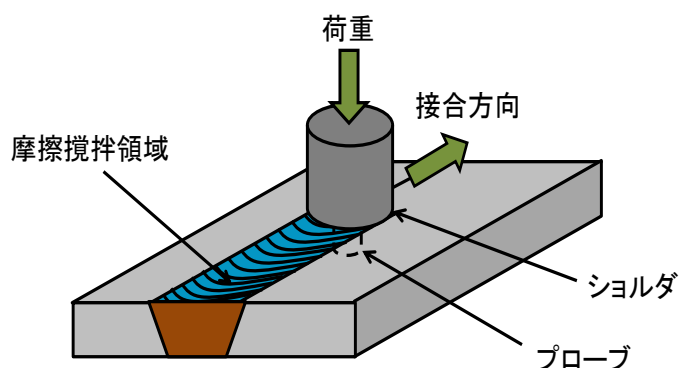
FSW(摩擦攪拌接合)の模式図
